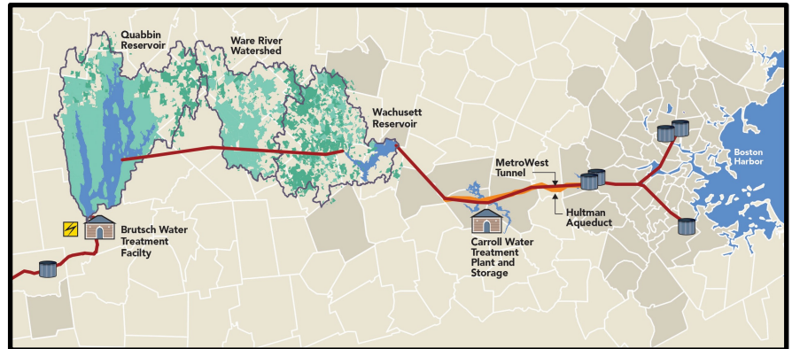
MWRA输水隧道系统
